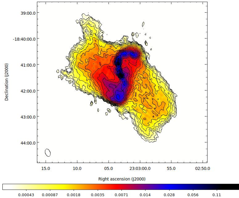
uGMRT 400 MHz map
